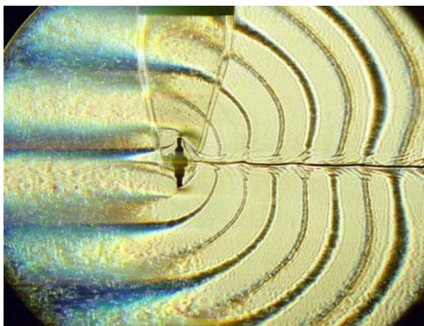
Волны, вихри и лигаменты в стратифицированном течении за пластиной
